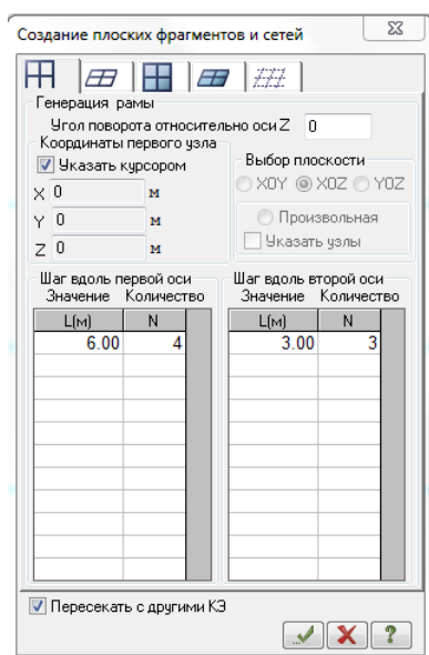
Рис.1 Создание геометрической схемы рамы
