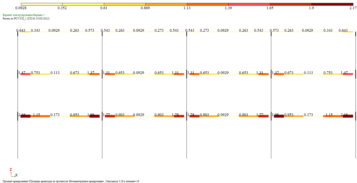
Рис.7 Расчетное армирование ригелей
